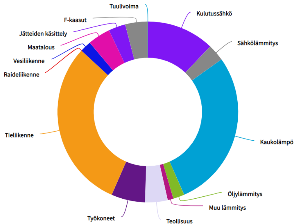
Uudenmaan päästöjakauma 2021
